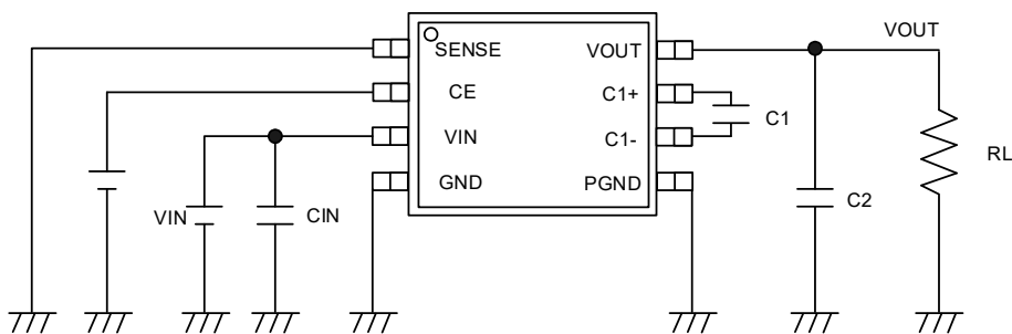
CIRCUIT④
