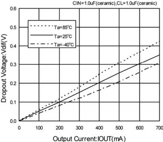
XC6210 (VOUT:3.0V)
