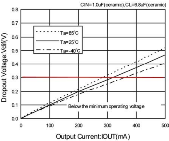
XC6210 (VOUT:1.2V)
