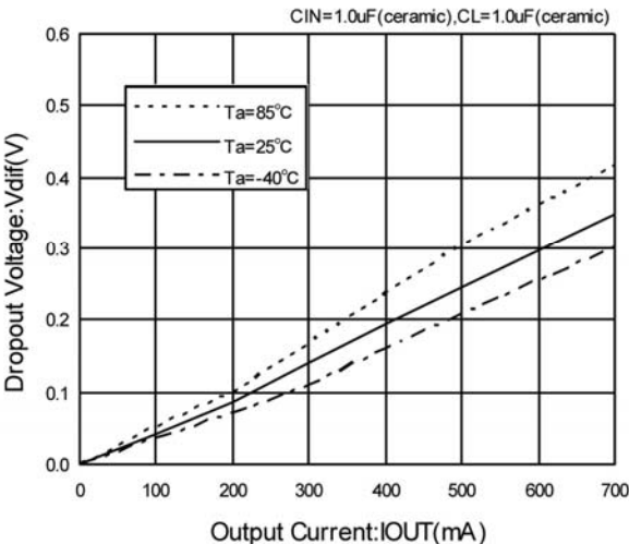
XC6210 (VOUT:5.0V)
