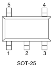
SOT-25
