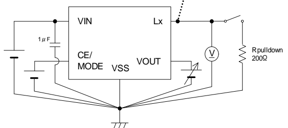
Circuit④
