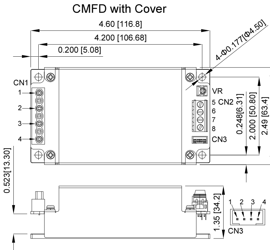
CN1 & CN2 PIN CONNECTION
