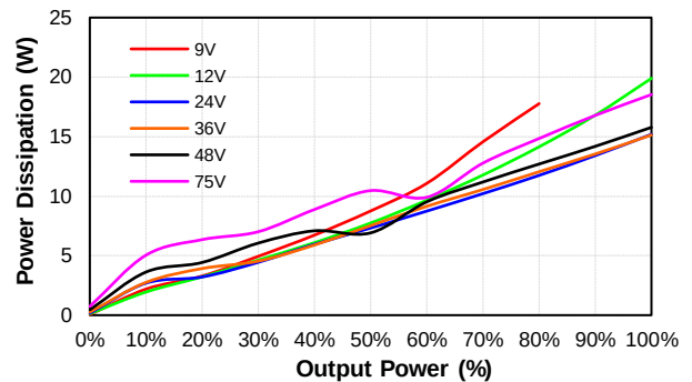
CQB150W8-36S28 Pd Vs Po @25 Deg. C
