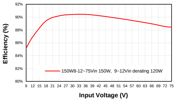
CQB150W8-36S54 Eff Vs Vin @25 Deg. C
