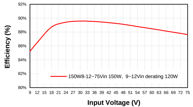
CQB150W8-36S24 Eff Vs Vin @25 Deg. C
