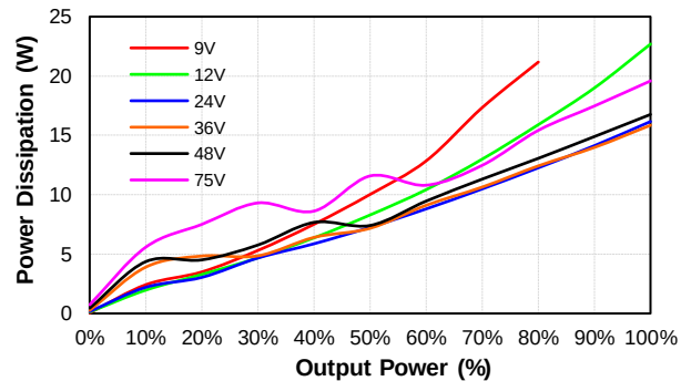
CQB150W8-36S54 Pd Vs Po @25 Deg. C
