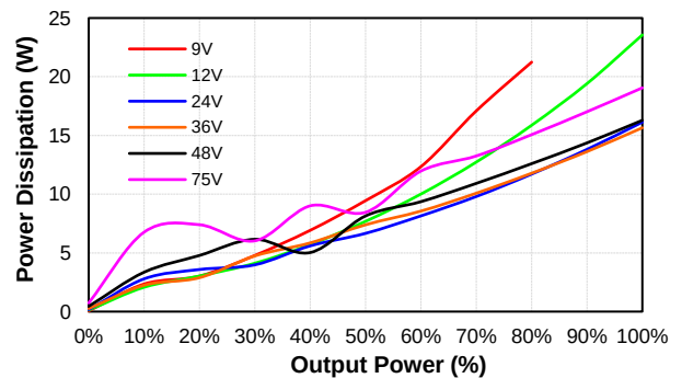
CQB150W8-36S12 Pd Vs Po @25 Deg. C
