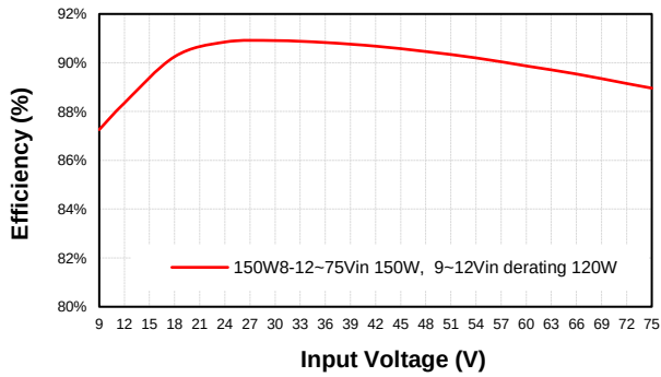
CQB150W8-36S28 Eff Vs Vin @25 Deg. C
