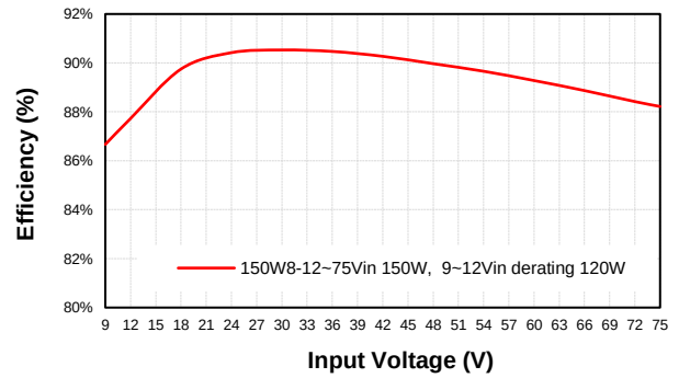
CQB150W8-36S48 Eff Vs Vin @25 Deg. C
