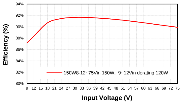
CQB150W8-36S15 Eff Vs Vin @25 Deg. C
