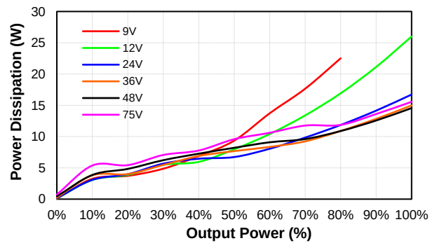
CQB150W8-36S05 Pd Vs Po @25 Deg. C
