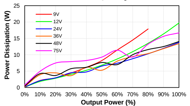
CQB150W8-36S15 Pd Vs Po @25 Deg. C
