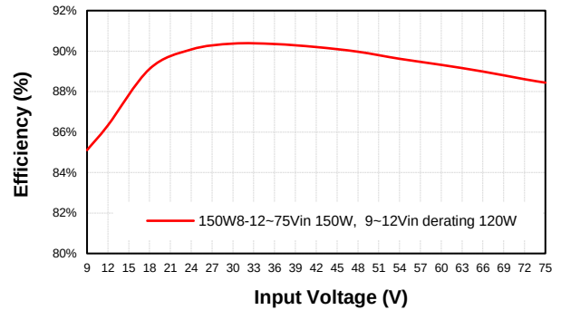
CQB150W8-36S12 Eff Vs Vin @25 Deg. C
