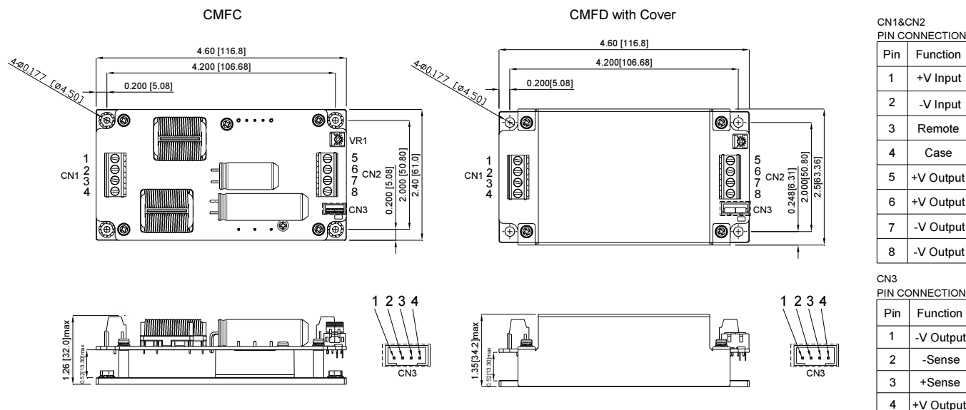
CQB50W12-72SXX-CMFC(D) Mechanical Outline Diagram
