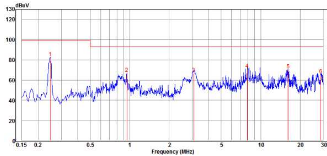
CQB50W12-72S12-CMFC
