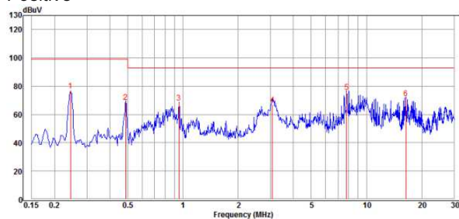
CQB50W12-72S48-CMFC
