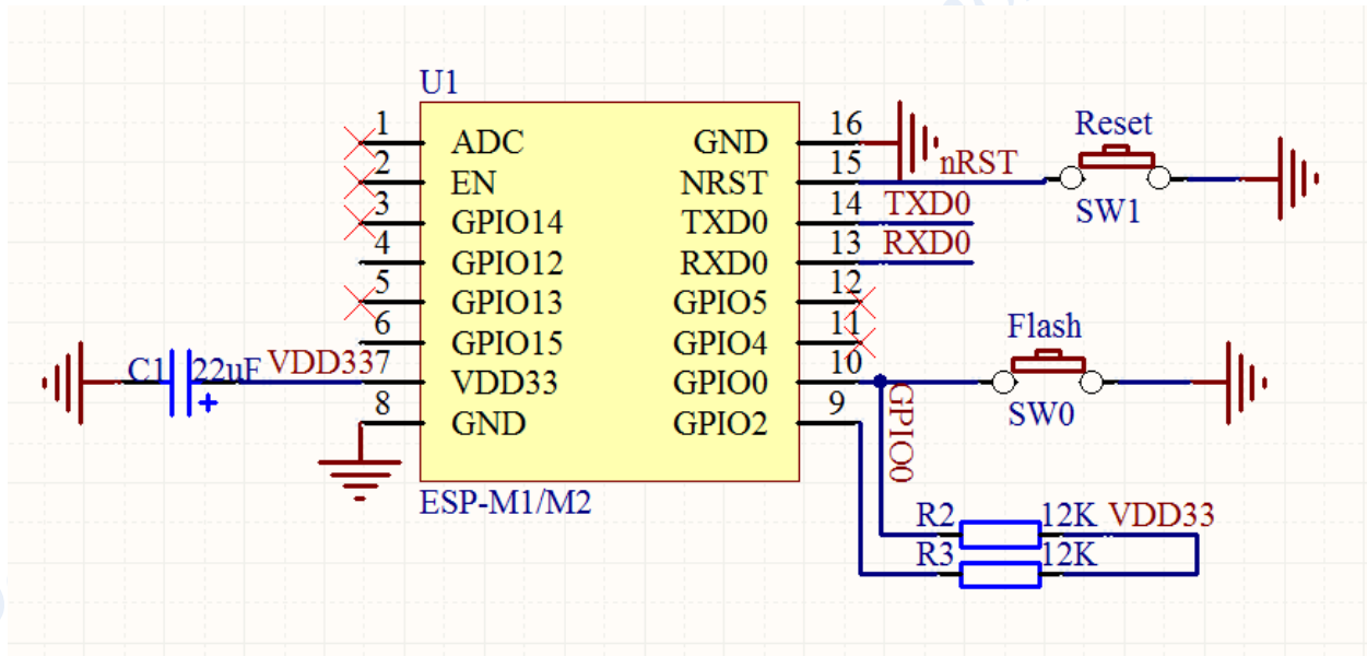
图 8.1 最小系统
