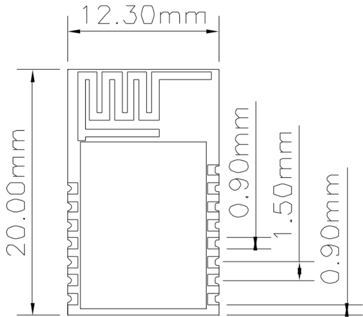
(a) 俯视图
