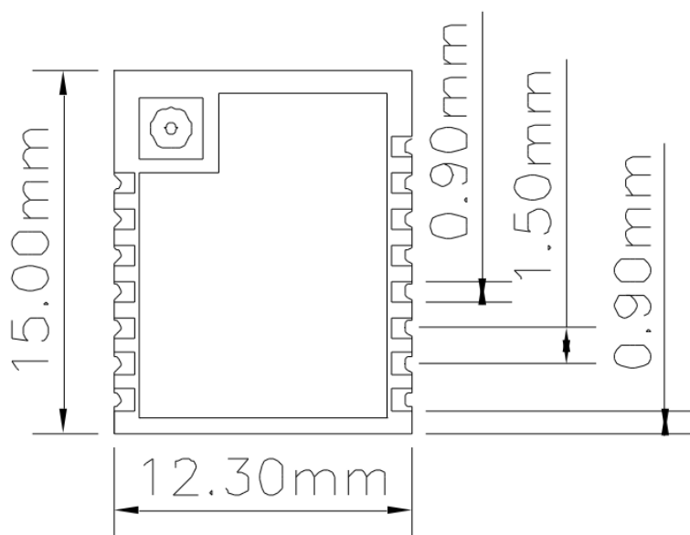
(a) 俯视图
