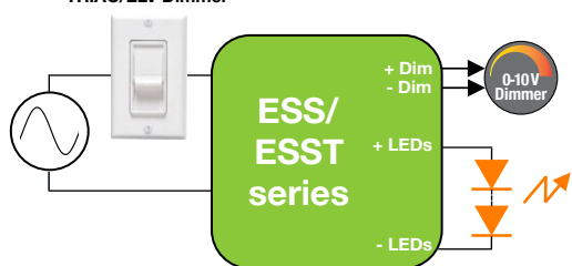
TRIAC/ELV Dimmer
