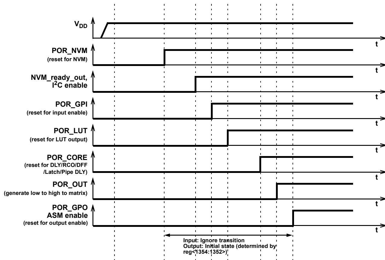
Figure 73. POR sequence
