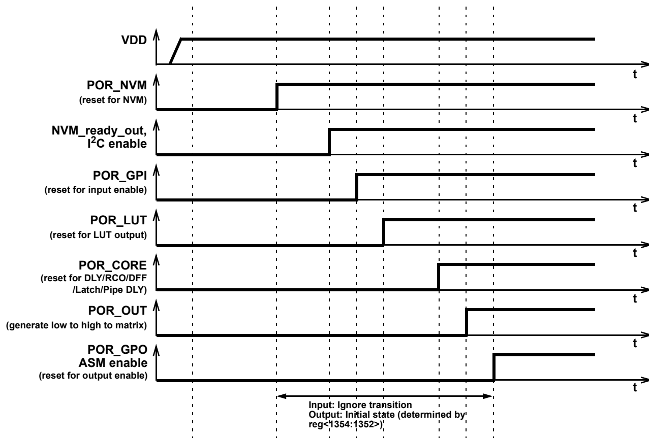
Figure 61. POR sequence
