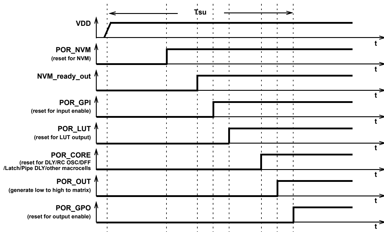
Figure 43. POR sequence
