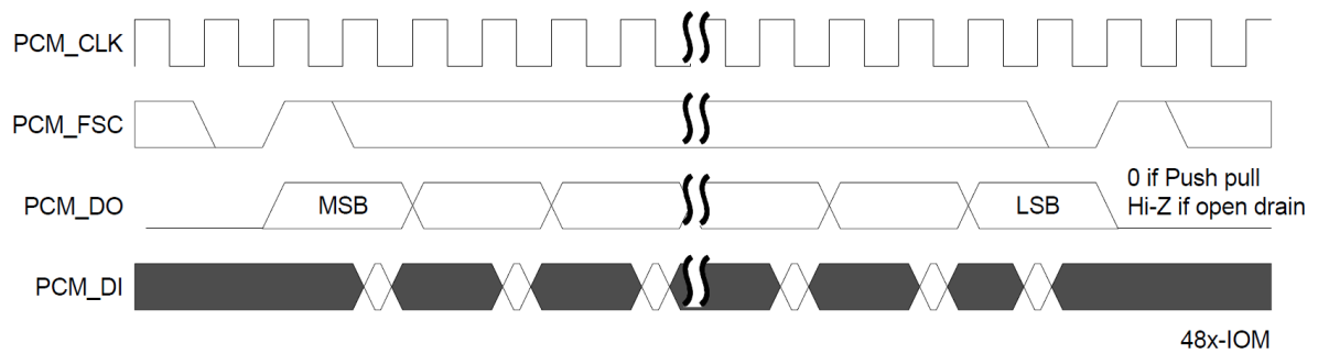
Figure 71: IOM format
