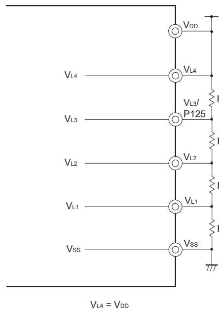
(d) 1/4 bias method
