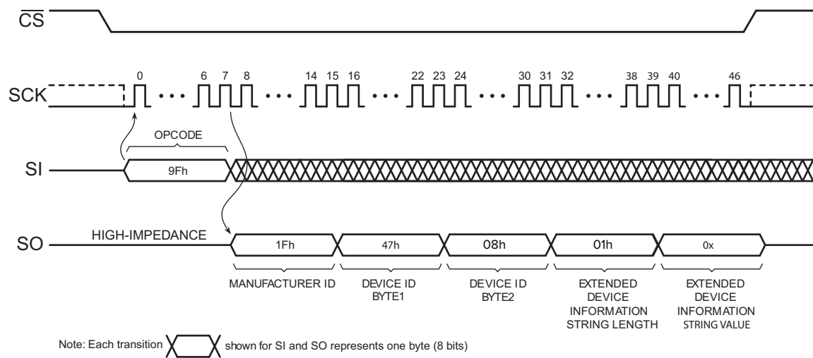
Figure 7-7. Read JEDEC ID
