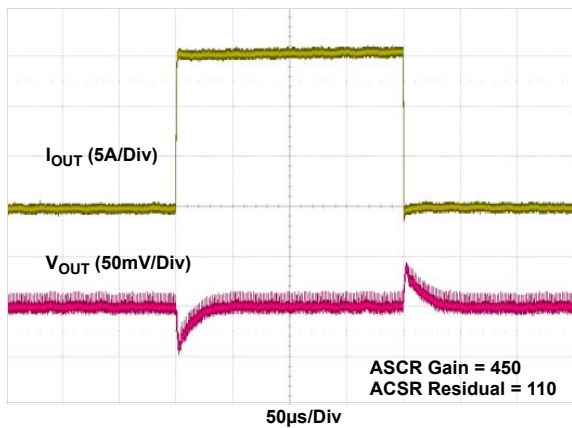
Figure 29. 0A - 15A, 12V_{IN} , 1V_{OUT} , 615kHz
