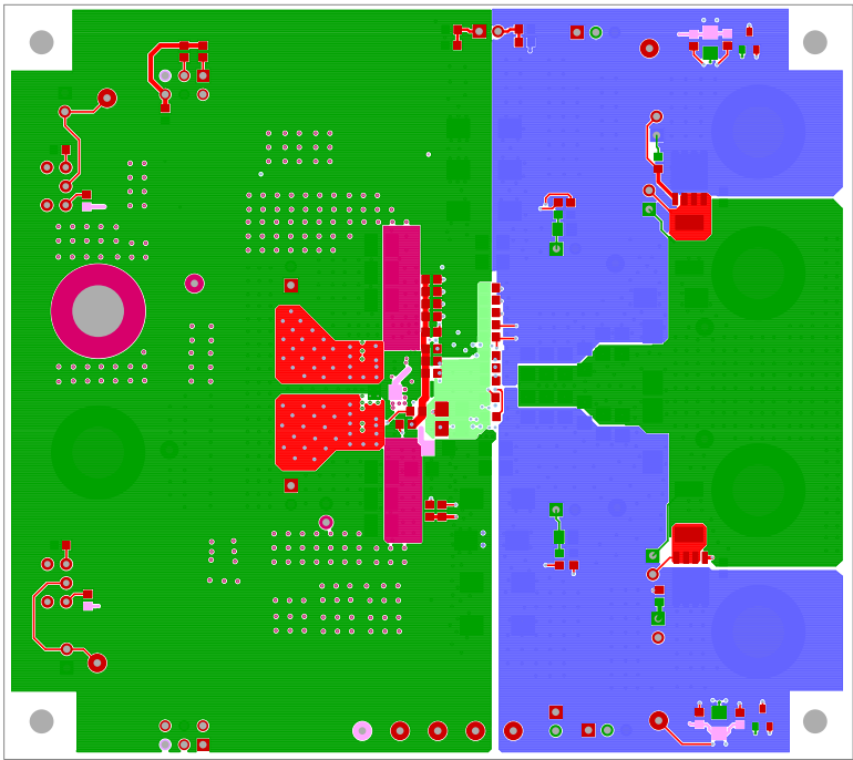
Figure 19. Bottom Layer
