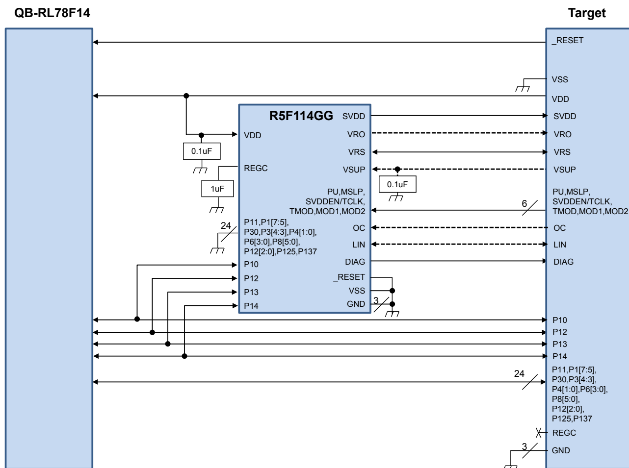
図1-3 QB-R5F114GG-EA-01T構成図
