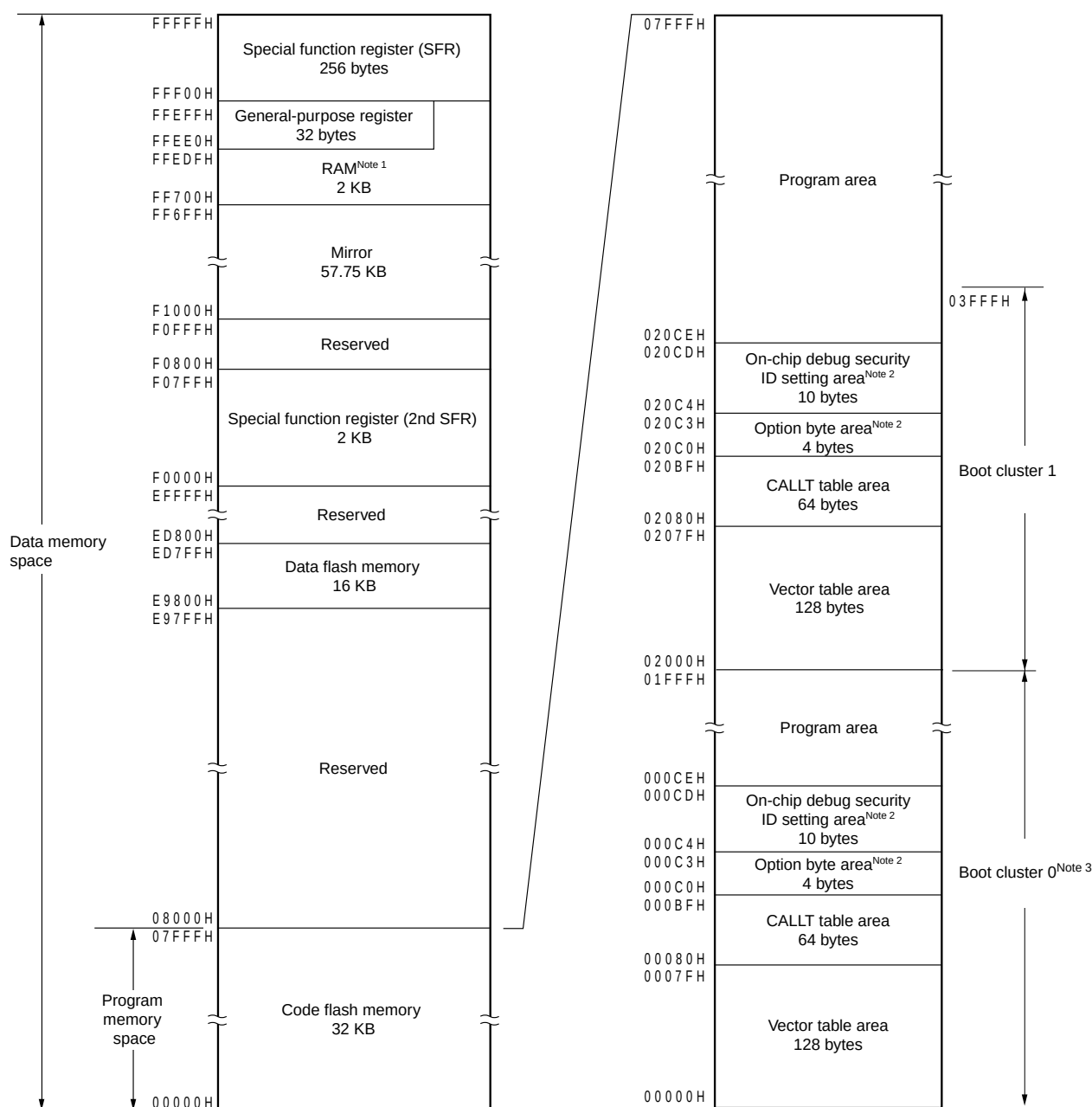
Figure 3-2. Memory Map (μPD78F1805, 78F1809, 78F1813, 78F1818)
