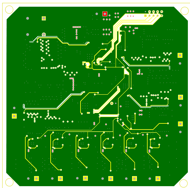
Figure 20. Bottom Layer
