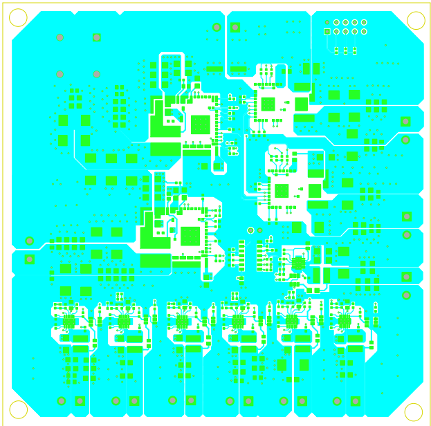
Figure 17. Top Layer
