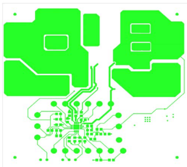
FIGURE 22. TOP LAYER
