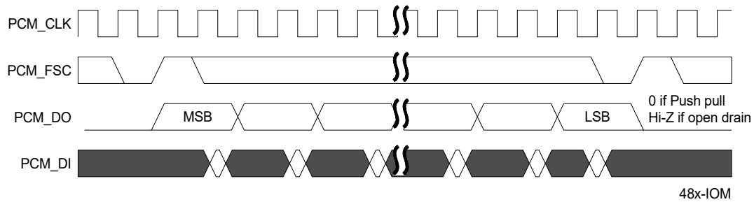
Figure 71: IOM format
