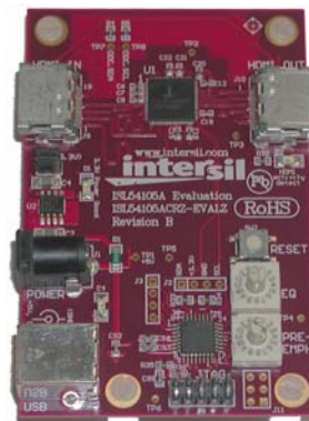
ISL54105A (1→1) ISL54105ACRZ-EVALZ
