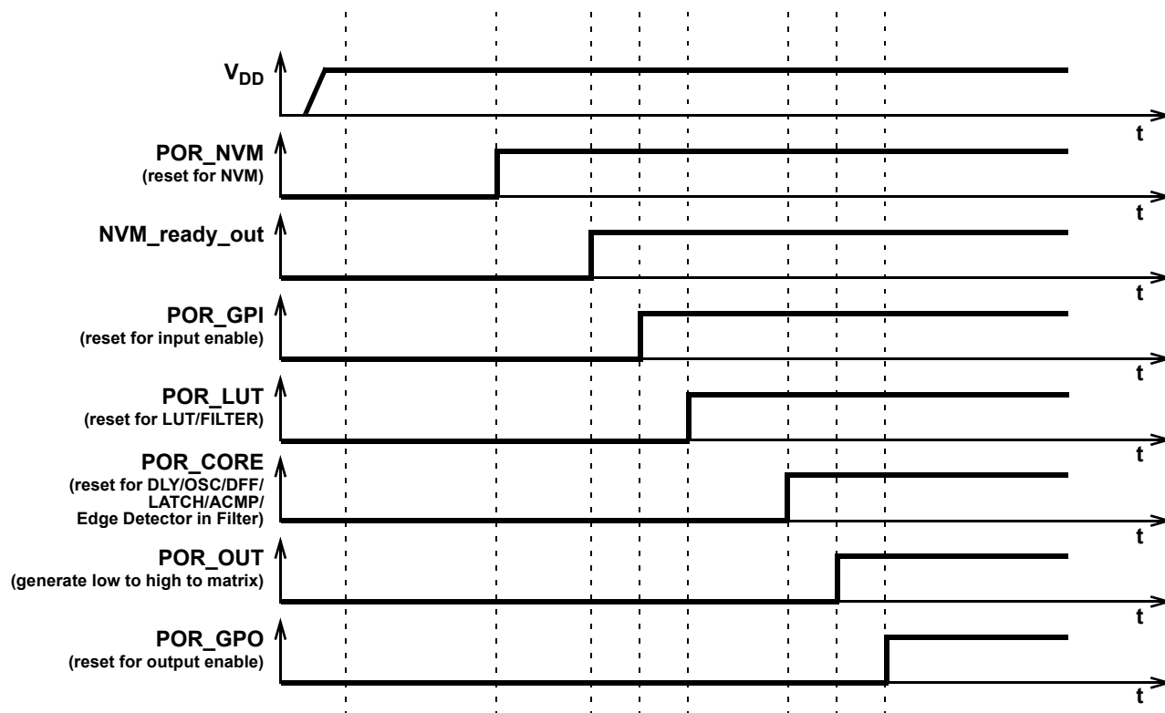
Figure 95: POR Sequence
