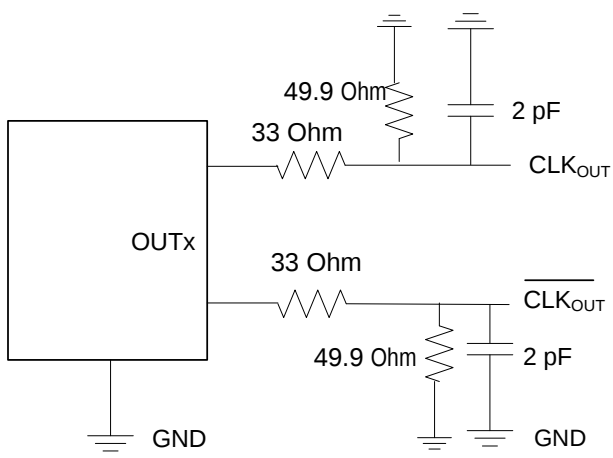
HCSL
