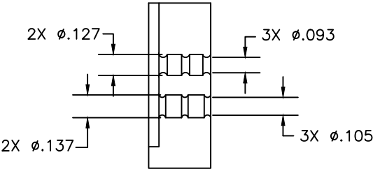
VIEW A-A
