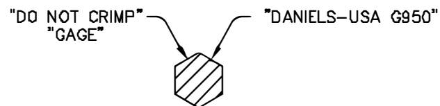
SECTION A-A
