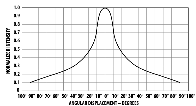
Figure 9: HLMP-Q102/-Q152
