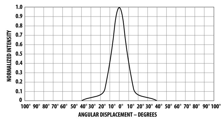
Figure 8: HLMP-Q106/-Q156
