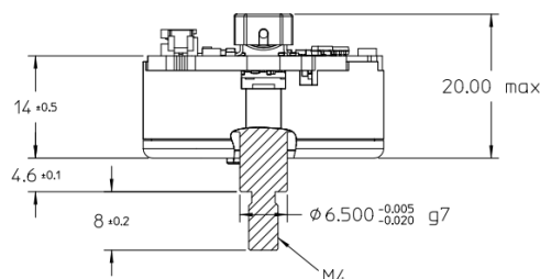
M4 Hub Screw
