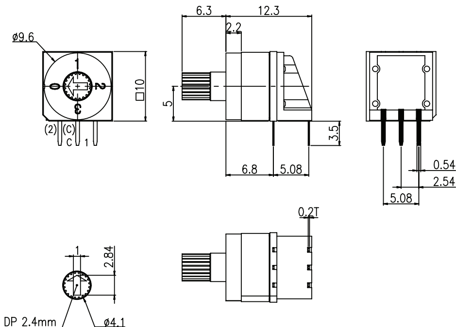
ACTUATOR
