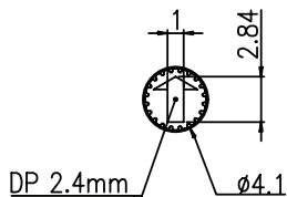
ACTUATOR
