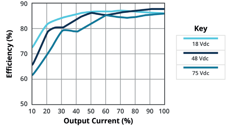
EFFICIENCY VS OUTPUT LOAD PDQ15-Q48-D15-D
