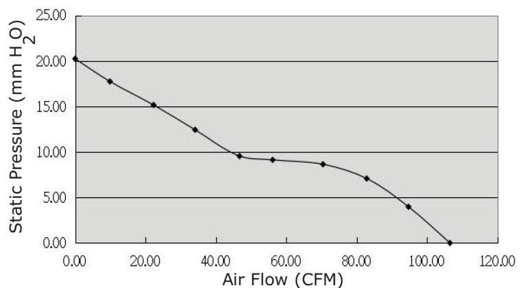
CFM-9225BG68-257-533
