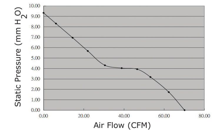
CFM-9225BG68-257-533
