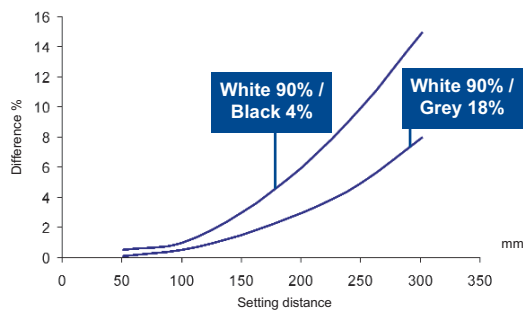
Background suppression
