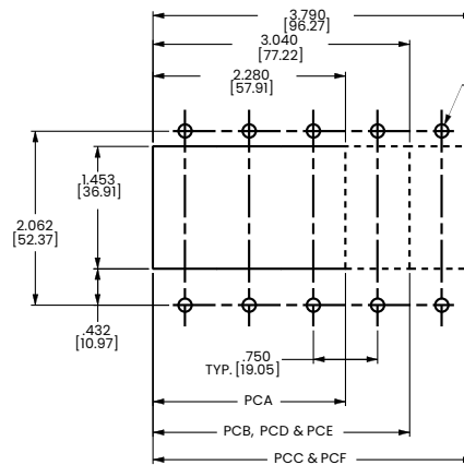
HANDLE ACTUATOR
