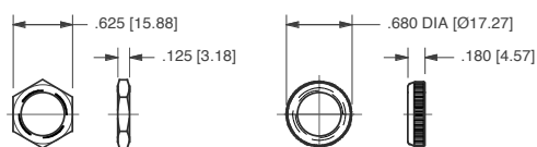
HEX NUT
