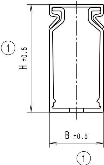
Montagezustand mit Deckel/ Assembled with cover
