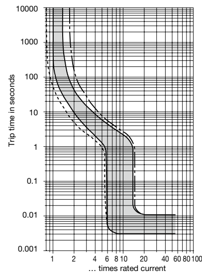
-T1 0.05...6 A
