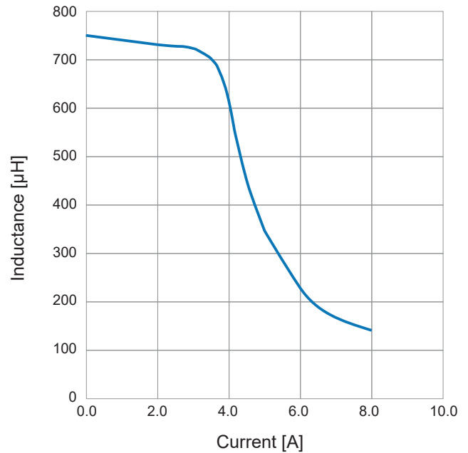
SPFC-RM10-50
