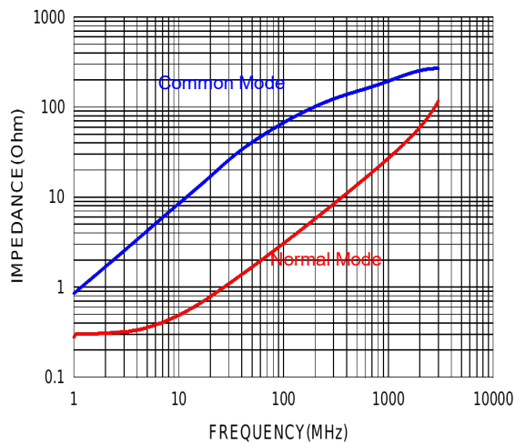
SPDL2012-670-2P-T
