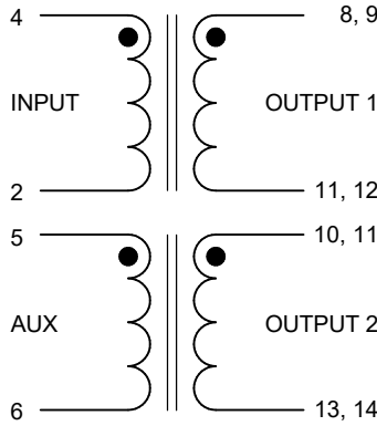
SLLC-ETD39
