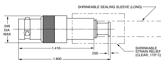
CJ70C-202 Shown
