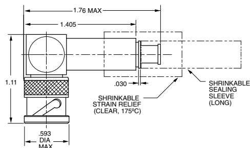
PLR74C-201 Shown
