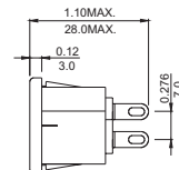
SOLDER LUG
