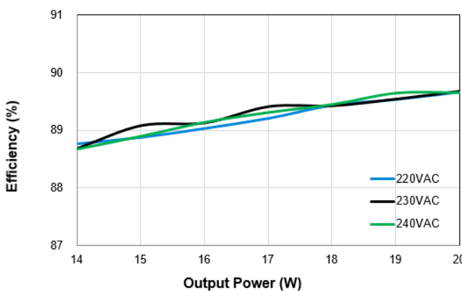
LNP-07A20WBCA – 700mA
