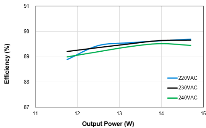
LNP-03A20WBCA – 350mA
