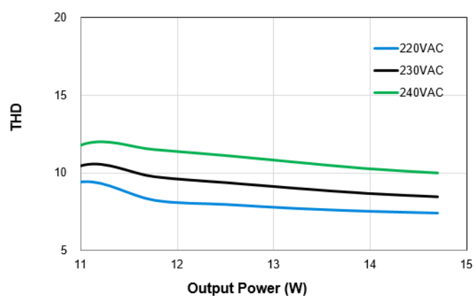
LNP-03A20WBCA – 350mA
