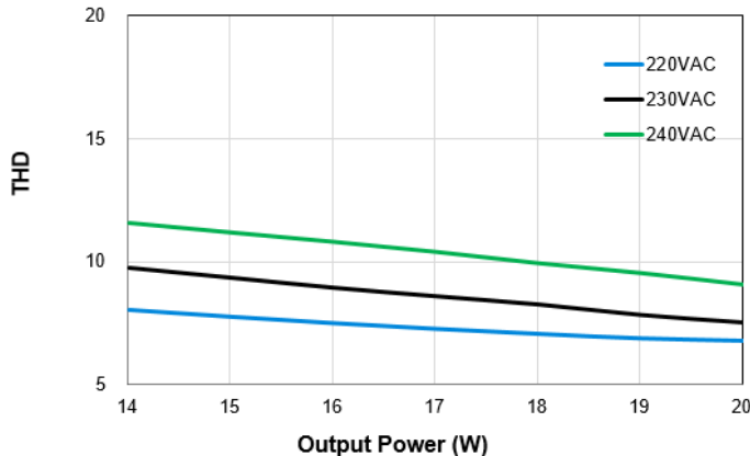
LNP-07A20WBCA – 700mA
