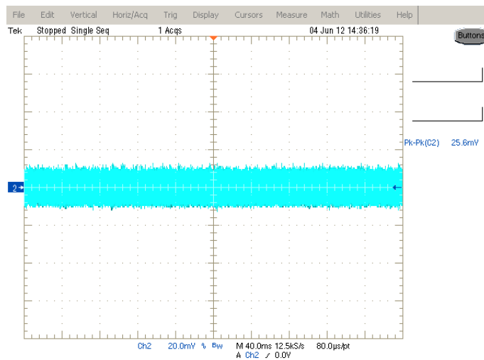
(b) 230 V
