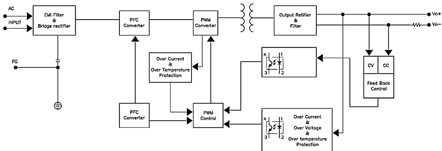
LNE-□V185WD□□
