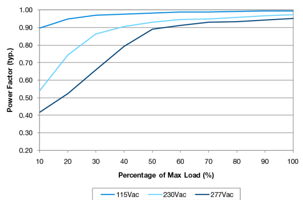
LNE-48V150W□
