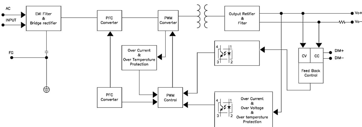
LNE-□V120WD□□□
