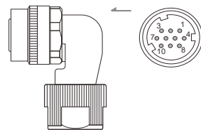
ACS3-CNEN2C00 (for F100 - F180) Mil-Spec: CMV1-AP10S
