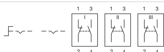
Wiring diagram 122
