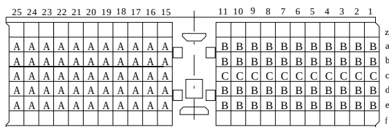
Bestückungsplan - contact layout
