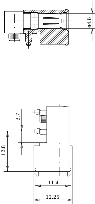
Federleisteengehäuse - Female housing 114939
