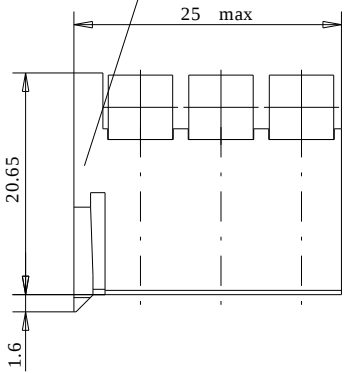
Federleisteengehäuse - Female housing 114939
