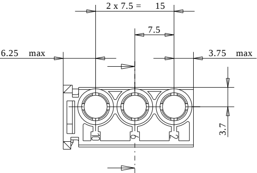
Federleisteengehäuse - Female housing 114939
